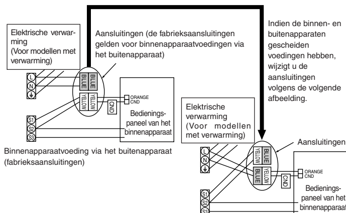
Gescheiden binnen-/buitenapparaatvoedingen
