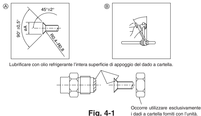
① Dimensioni di taglio per raccordo a cartella
