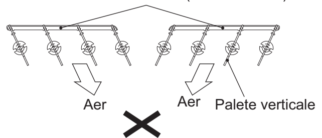
Unitatea lamei verticale (vedere de sus)
