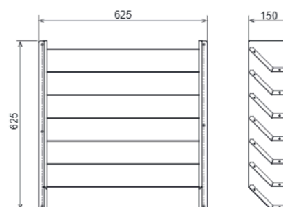
PAC-SH96SG-E
