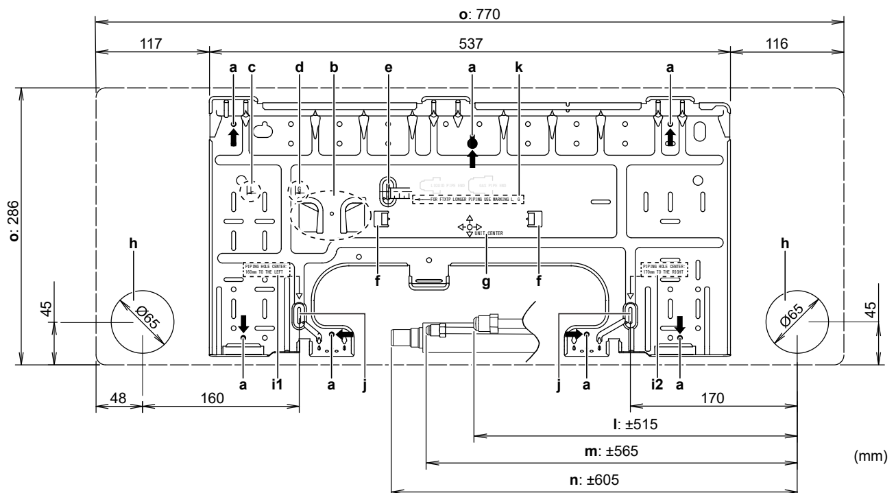
a Locuri de fixare recomandate pentru placa de montare b Buzunar pentru capacul orificiului conductei c Capătul conductei de lichid d Capătul conductei de gaz e Folosiți ruleta așa cum este prezentat f Urechi pentru plasarea unei nivele cu bulă de aer g Centrul unității h Orificiu pentru tubulatura încăstrată Ø65 mm
